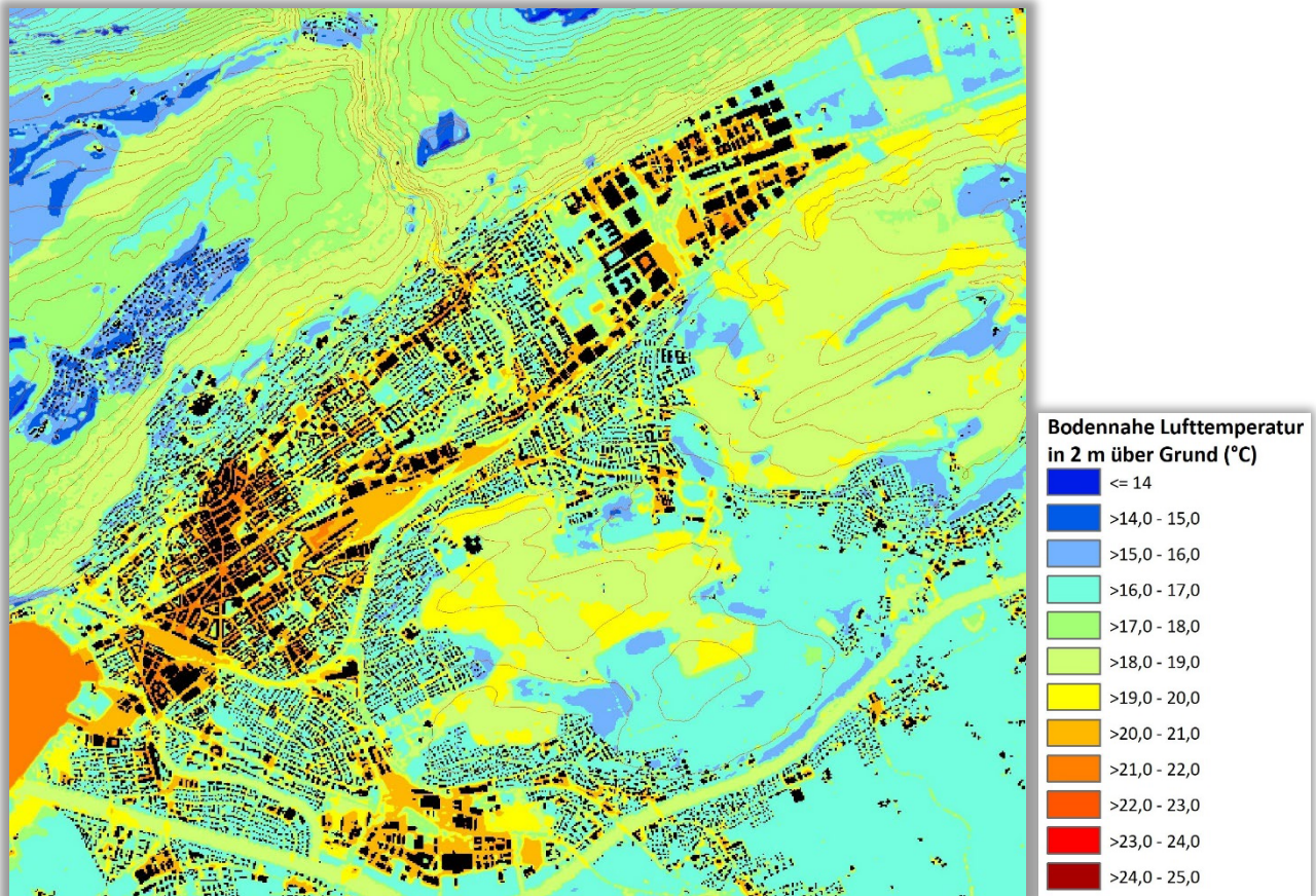
Abb. 4.1: Temperaturfeld Gegenwart im Bereich Biel zum Zeitpunkt 4 Uhr morgens (2m ü. Grund)
