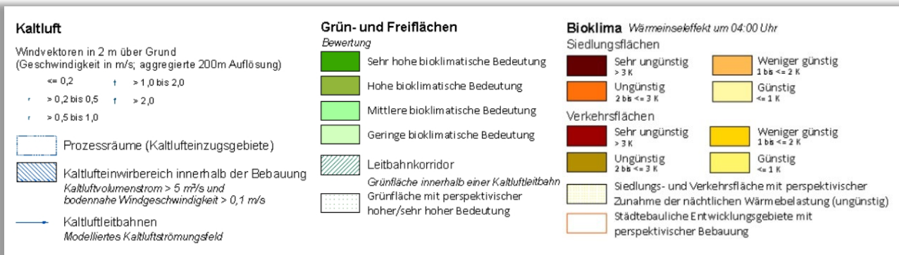
Abb. 7.3: Planungshinweiskarte Nacht mit Entwicklungsflächen im Raum Bern
