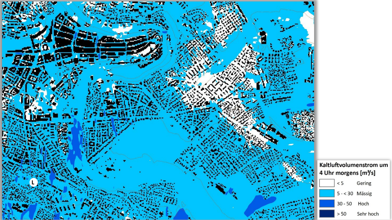
Abb. 4.26: Kaltluftvolumenstrom Zukunftsszenario im Bereich Bern zum Zeitpunkt 4 Uhr
