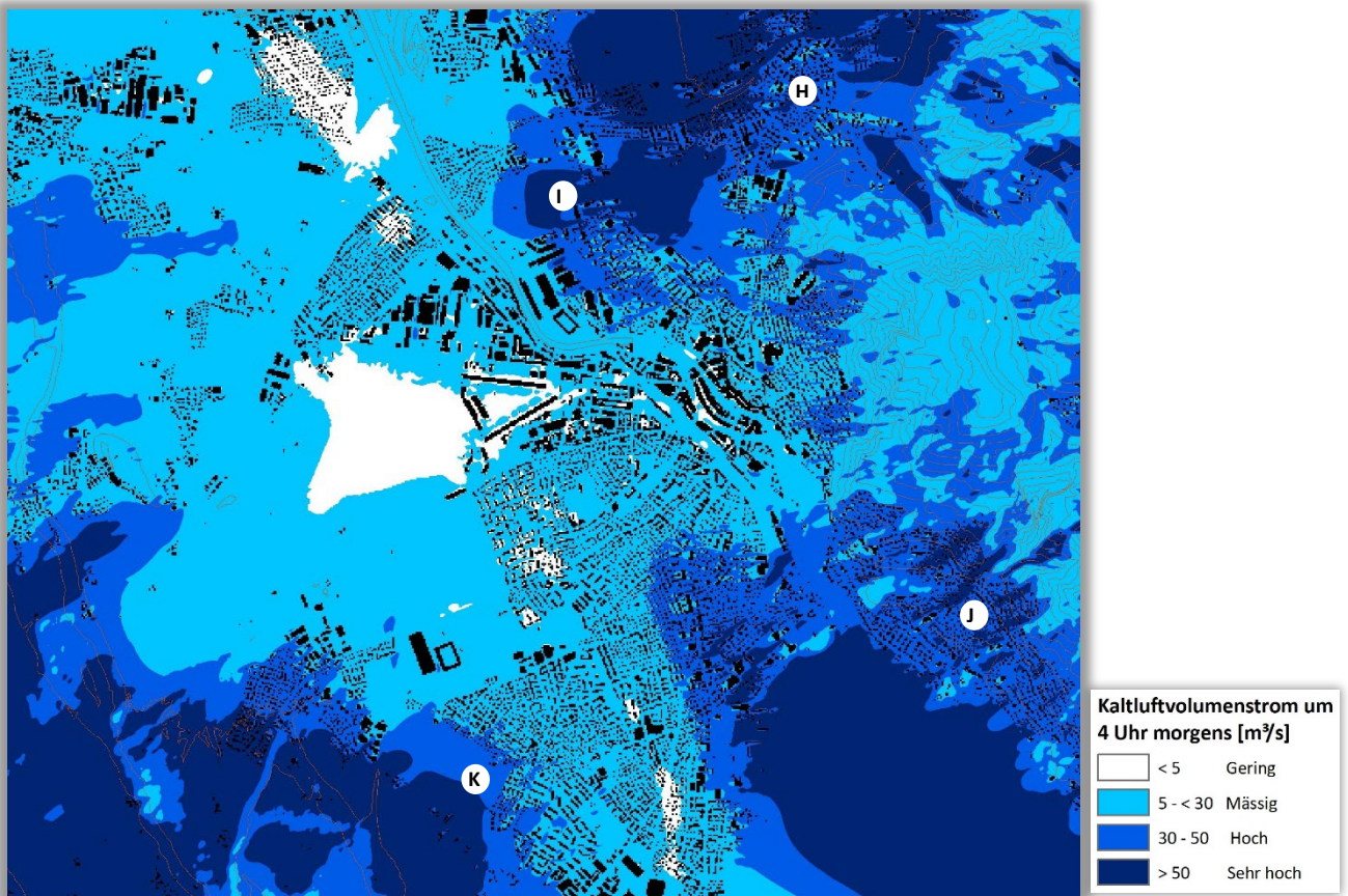
Abb. 4.24: Kaltluftvolumenstrom Gegenwart im Bereich Thun zum Zeitpunkt 4 Uhr
