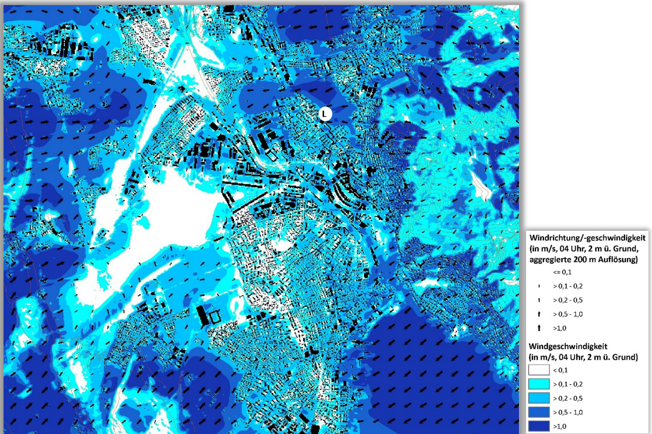
Abb. 4.19: Nächtliches Windfeld Zukunftsszenario im Bereich Thun zum Zeitpunkt 4 Uhr morgens (2m ü. Grund)
