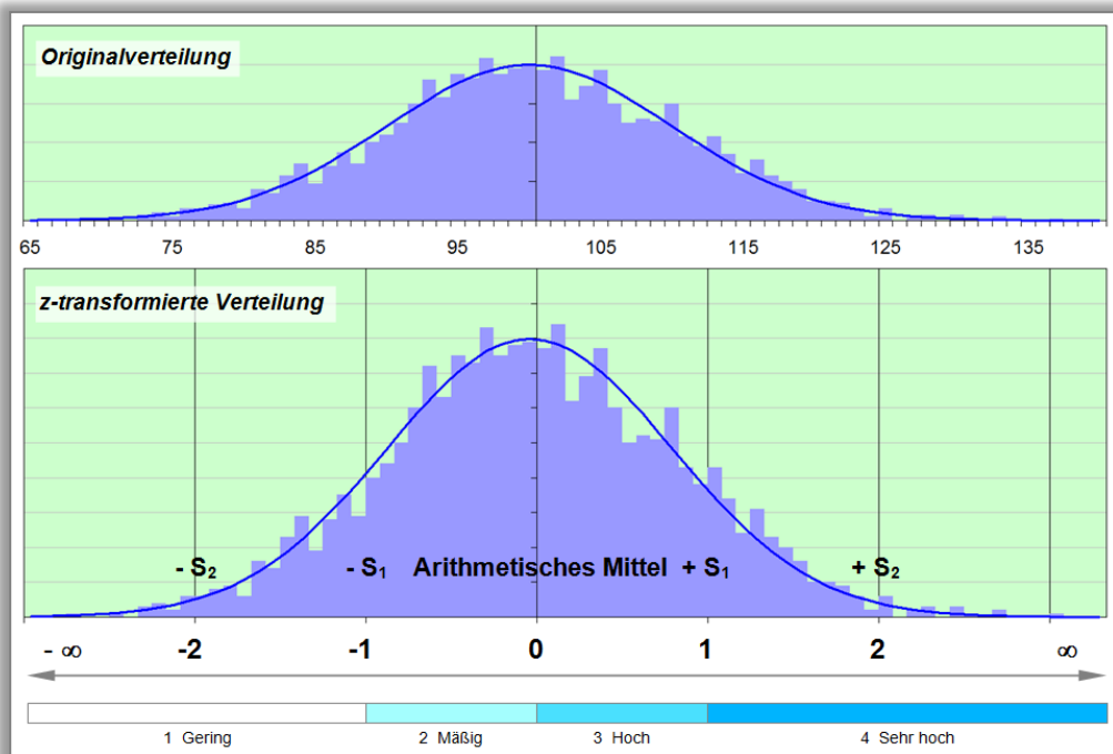
Abb. 4.21: Veranschaulichung der Standardisierung zur vergleichenden Bewertung von Parametern
