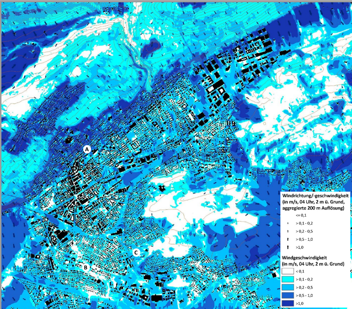
Abb. 4.14: Nächtliches Windfeld Gegenwart im Bereich Biel zum Zeitpunkt 4 Uhr morgens (2m ü. Grund)
