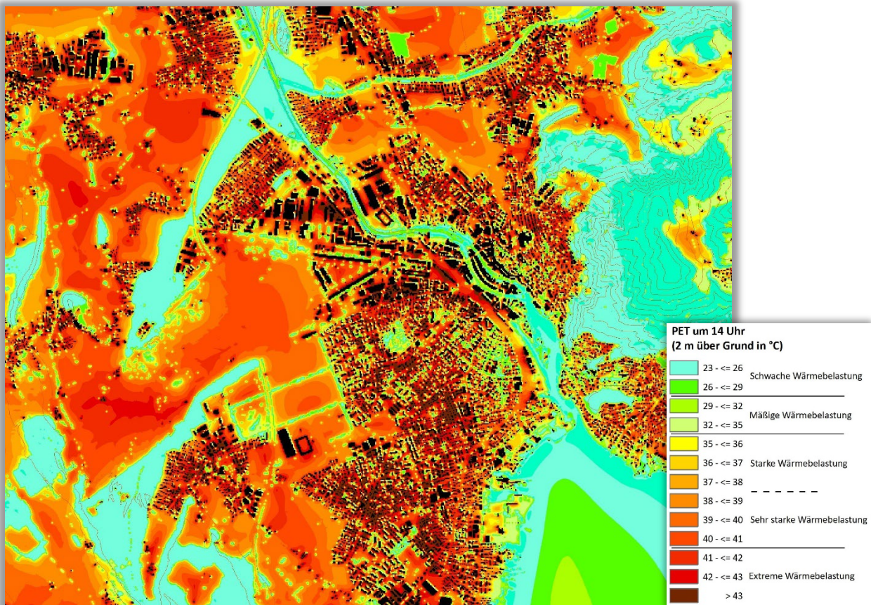
Abb. 4.9: PET Gegenwart im Bereich Thun zum Zeitpunkt 14 Uhr (2m ü. Grund)
