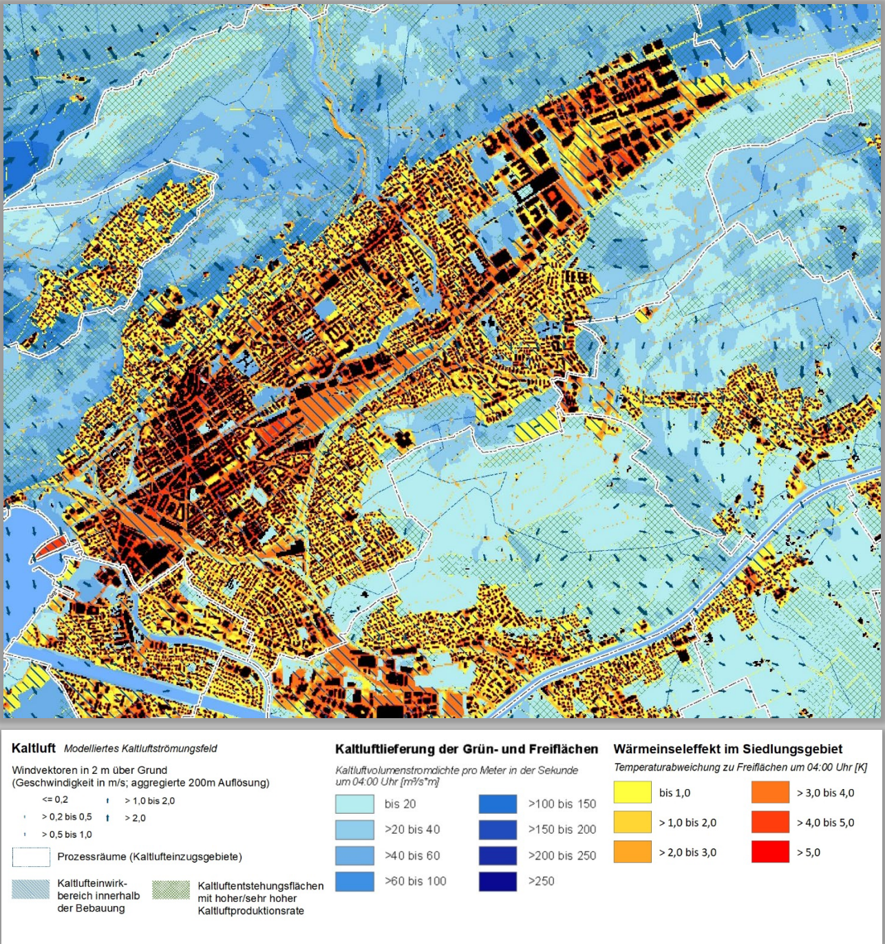
Abb. 5.1: Klimaanalysekarte im Bereich Biel - Gegenwart
