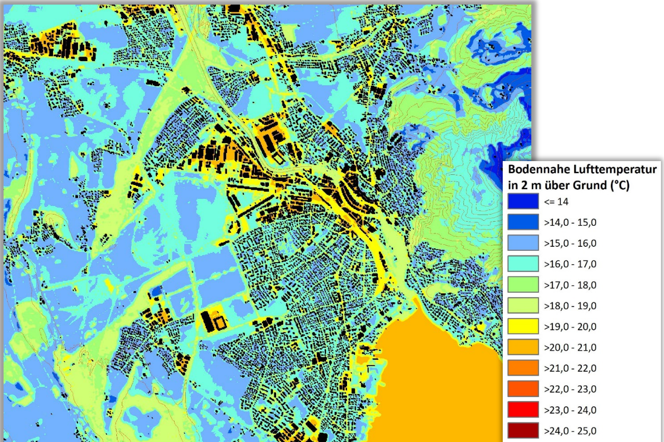
Abb. 4.3: Temperaturfeld Gegenwart im Bereich Thun zum Zeitpunkt 4 Uhr morgens (2m ü. Grund)
