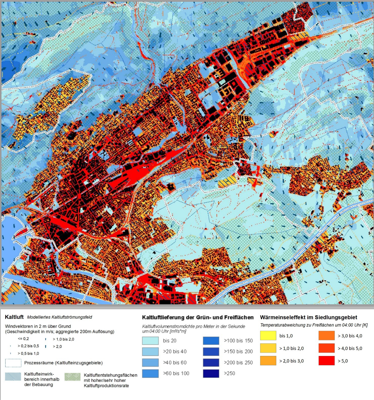
Abb. 5.2: Klimaanalysekarte im Bereich Biel – Zukunft
