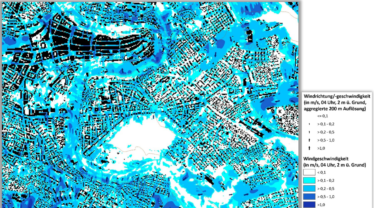
Abb. 4.18: Nächtliches Windfeld Zukunftsszenario im Bereich Bern zum Zeitpunkt 4 Uhr morgens (2m ü. Grund)
