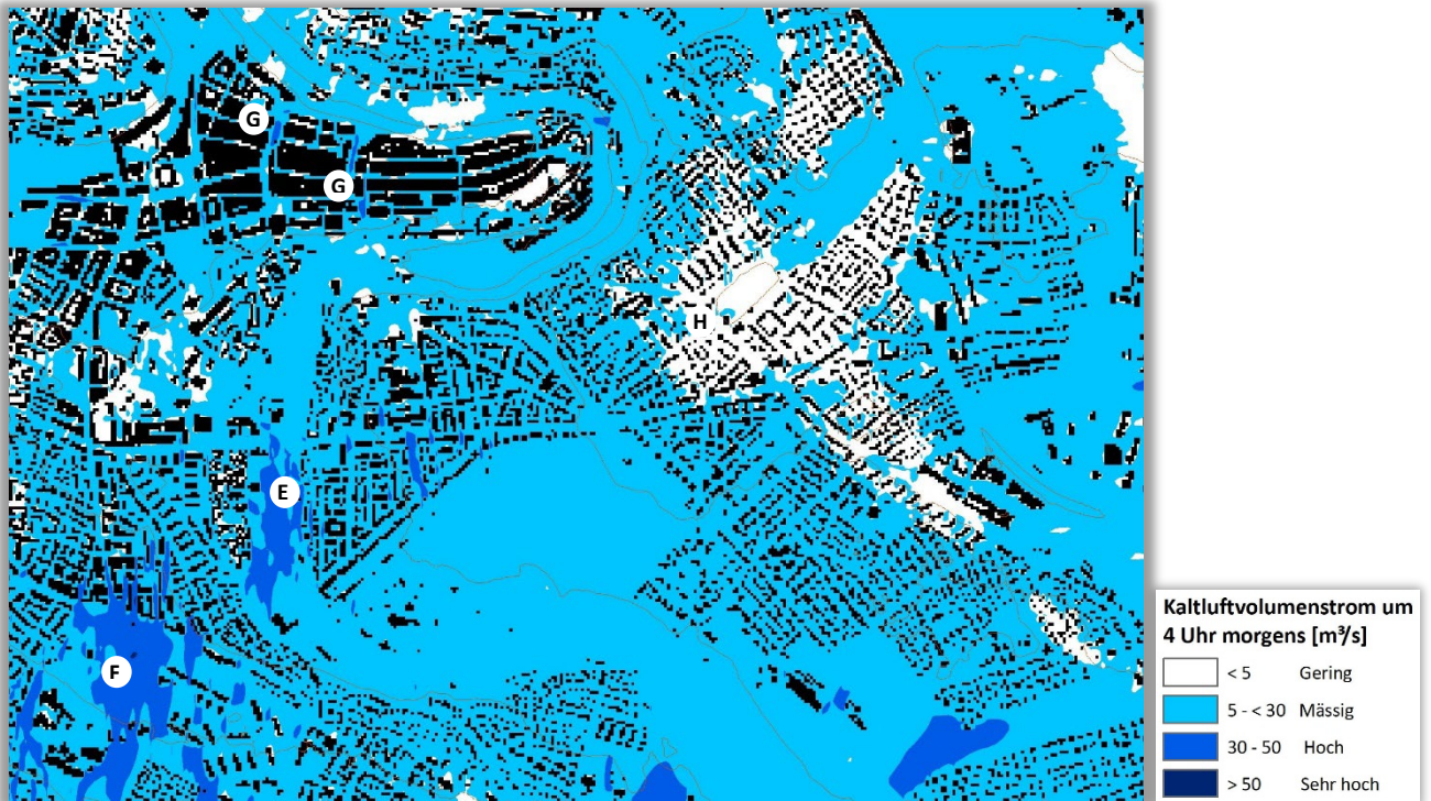
Abb. 4.23: Kaltluftvolumenstrom Gegenwart im Bereich Bern zum Zeitpunkt 4 Uhr morgens
