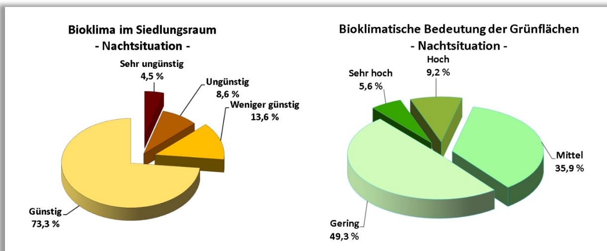
Abb. 6.3: Flächenanteile der bewerteten Nutzungsstrukturen im Kanton Bern (Nachtsituation) - Gegenwart
