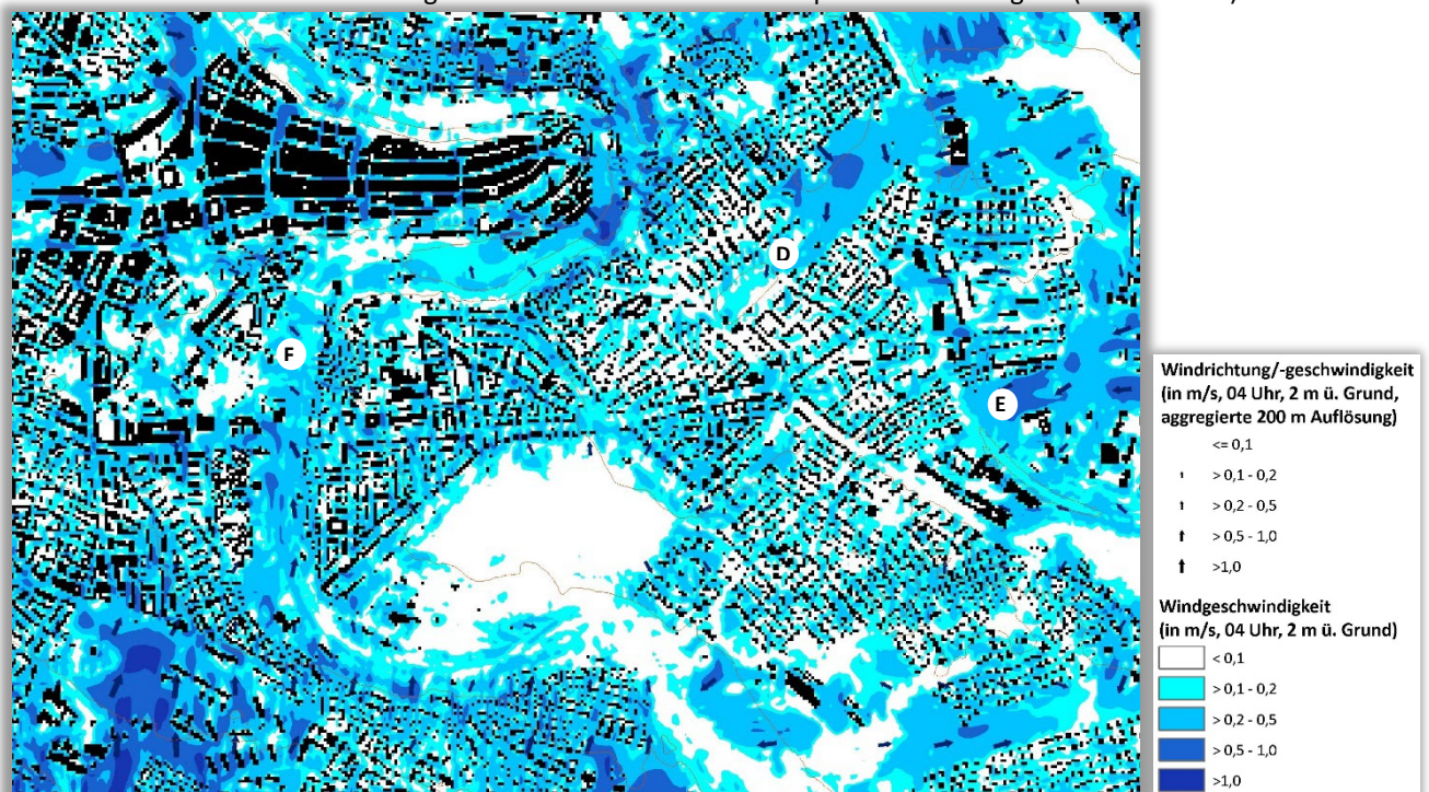
Abb. 4.15: Nächtliches Windfeld Gegenwart im Bereich Bern zum Zeitpunkt 4 Uhr morgens (2m ü. Grund)
