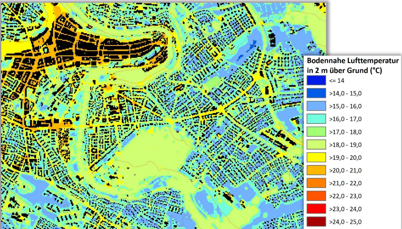
Abb. 4.2: Temperaturfeld Gegenwart im Bereich Bern zum Zeitpunkt 4 Uhr morgens (2m ü. Grund)
