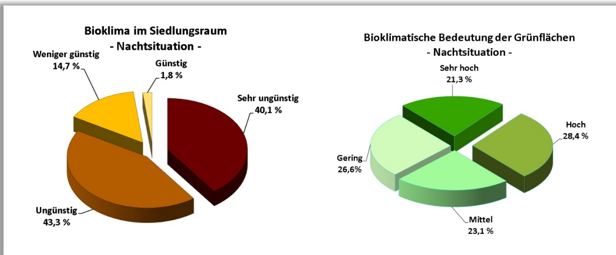
Abb. 6.4: Flächenanteile der bewerteten Nutzungsstrukturen im Kanton Bern (Nachtsituation) – Zukunft
