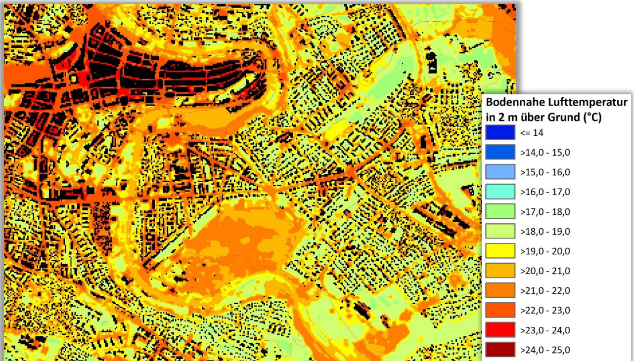
Abb. 4.5: Temperaturfeld Zukunftsszenario im Bereich Bern zum Zeitpunkt 4 Uhr morgens (2m ü. Grund)
