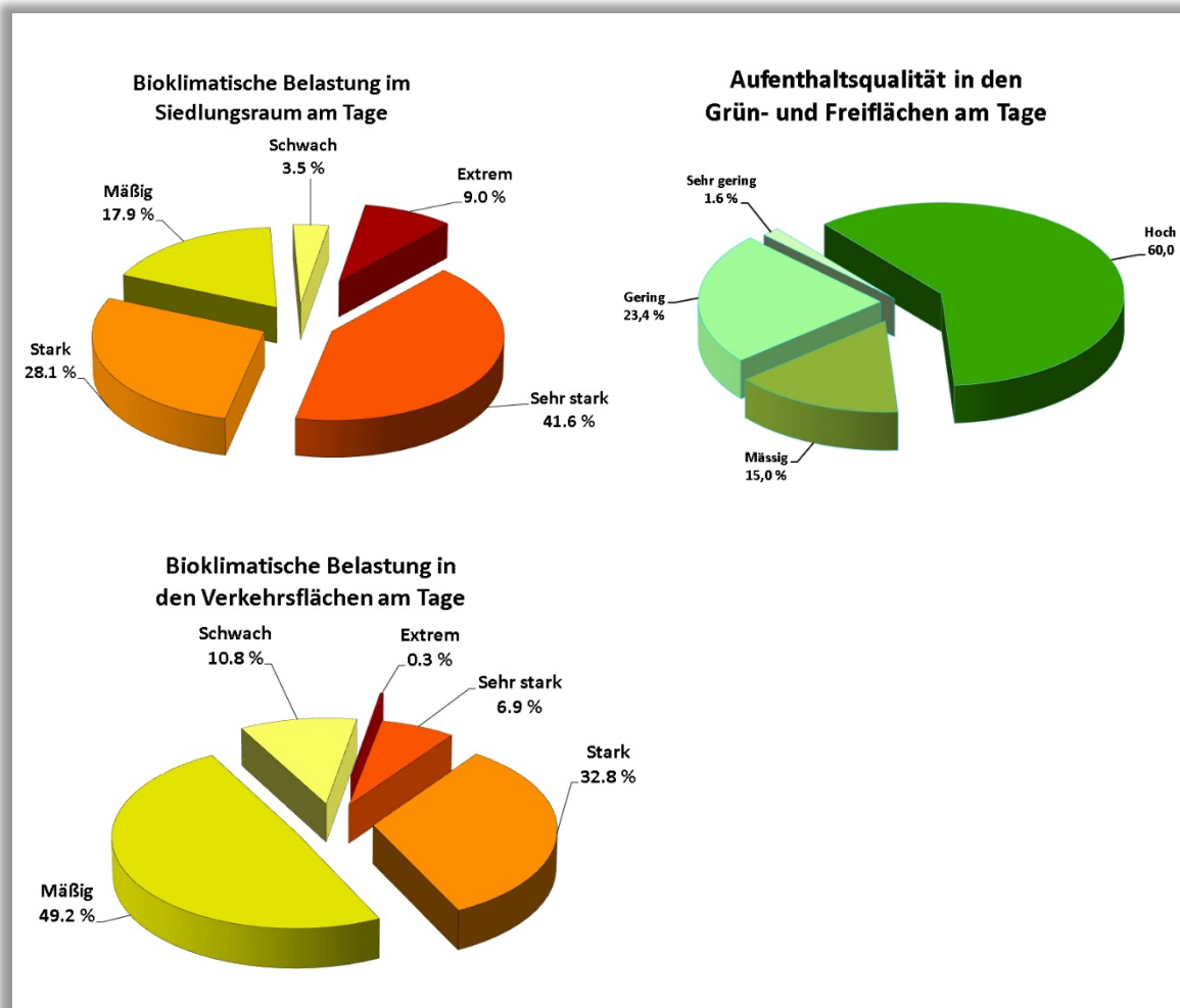
Abb. 6.6: Flächenanteile der bewerteten Nutzungsstrukturen im Kanton Bern (Tagsituation) - Gegenwart
