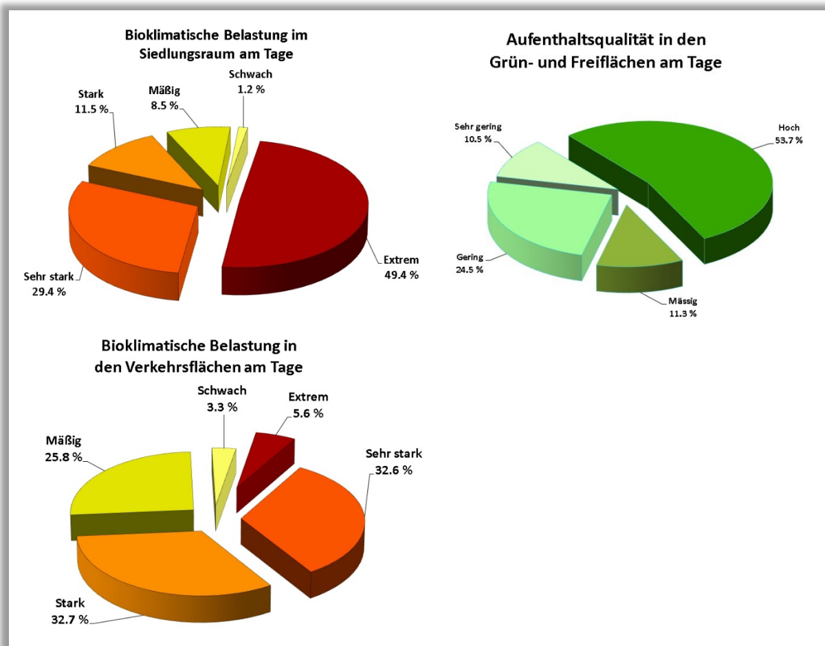
Abb. 6.8: Flächenanteile der bewerteten Nutzungsstrukturen im Kanton Bern (Tagsituation) - Zukunftsszenario
