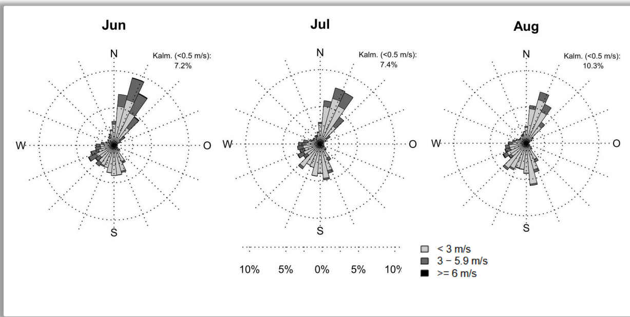
Abb. 3.7: Windrosen der Station Bern/Zollikofen 365 m ü.M. für die Sommermonate JJA. Quelle: (Meteoschweiz 2020c).
