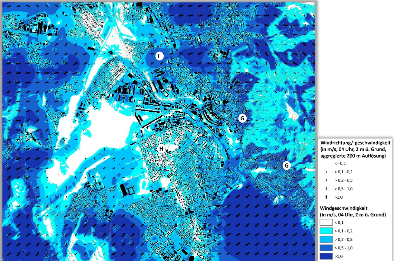
Abb. 4.16: Nächtliches Windfeld Gegenwart im Bereich Thun zum Zeitpunkt 4 Uhr morgens (2m ü. Grund)
