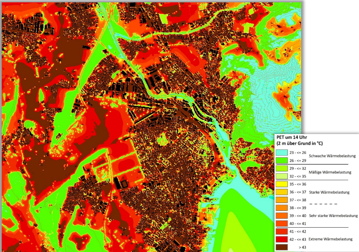
Abb. 4.12: PET Zukunftsszenario im Bereich Thun zum Zeitpunkt 14 Uhr (2m ü. Grund)
