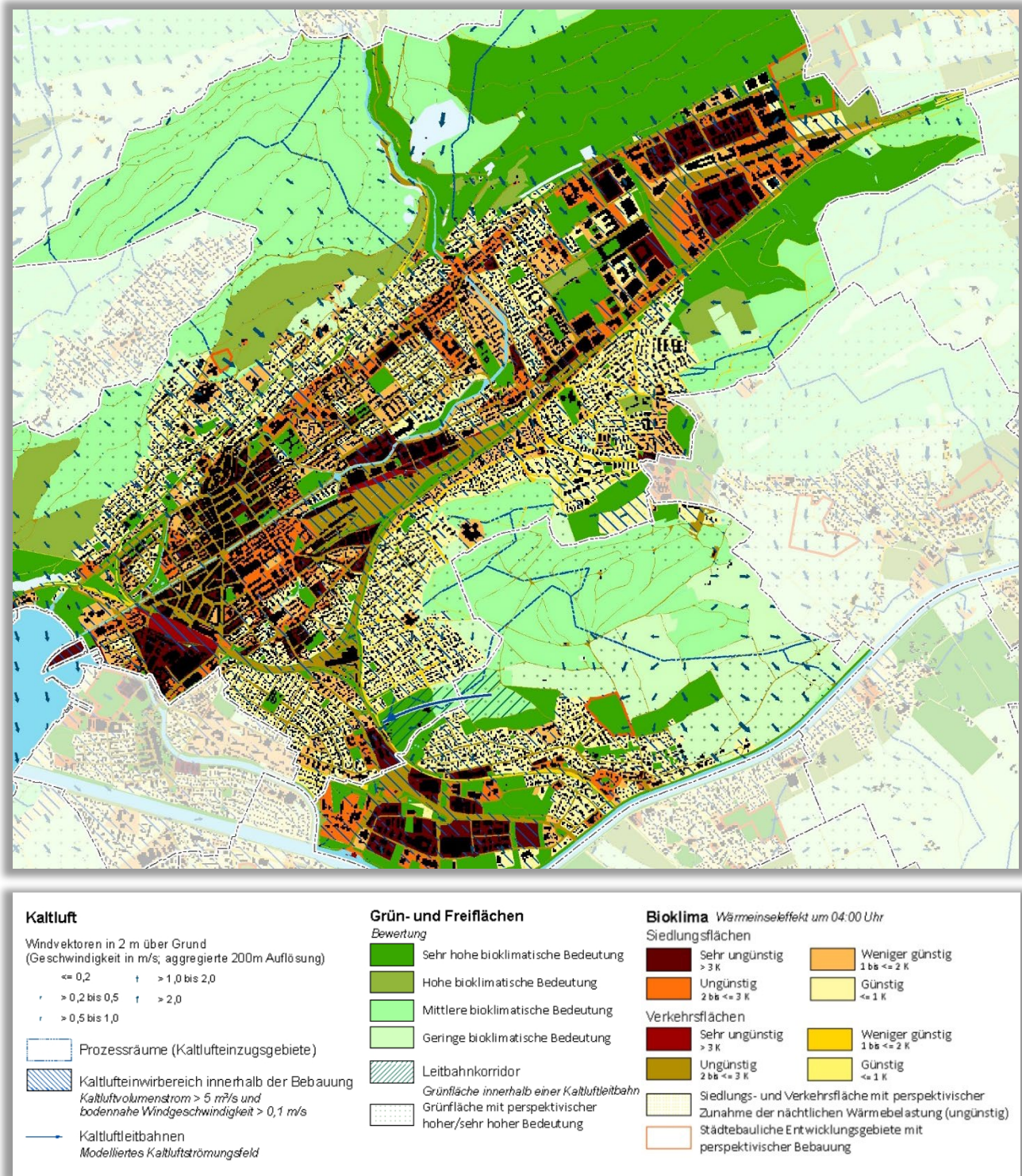
Abb. 6.2: Planungshinweiskarte Nachtsituation Gegenwart für den Bereich Biel
