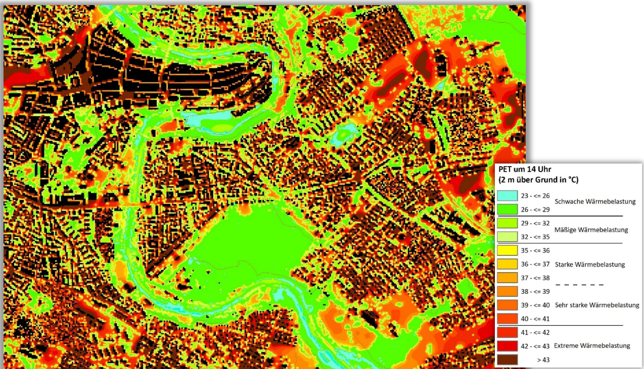
Abb. 4.11: PET Zukunftsszenario im Bereich Bern zum Zeitpunkt 14 Uhr (2m ü. Grund)
