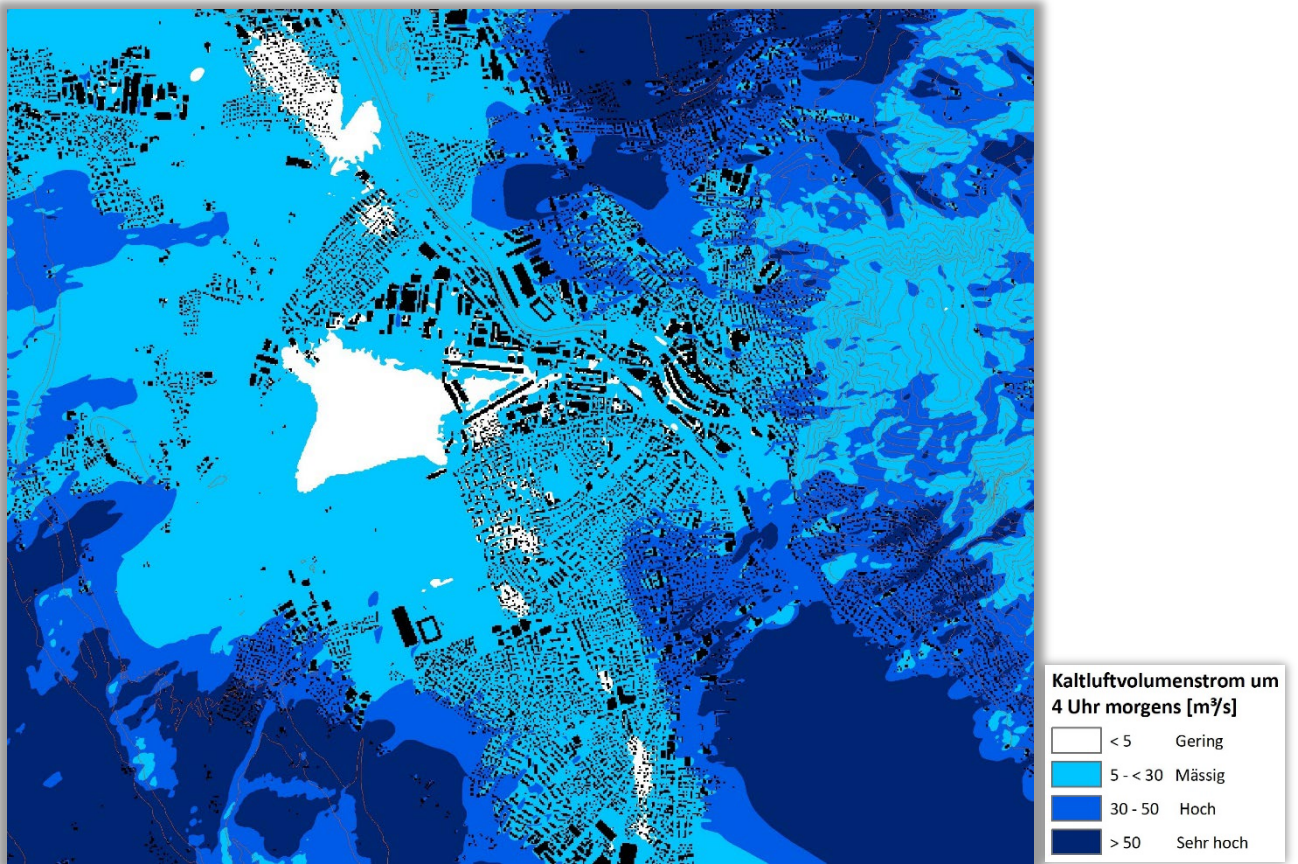
Abb. 4.27: Kaltluftvolumenstrom Zukunftsszenario im Bereich Thun zum Zeitpunkt 4 Uhr
