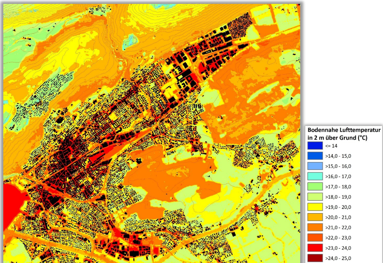
Abb. 4.4: Temperaturfeld Zukunftsszenario im Bereich Biel zum Zeitpunkt 4 Uhr morgens (2m ü. Grund)
