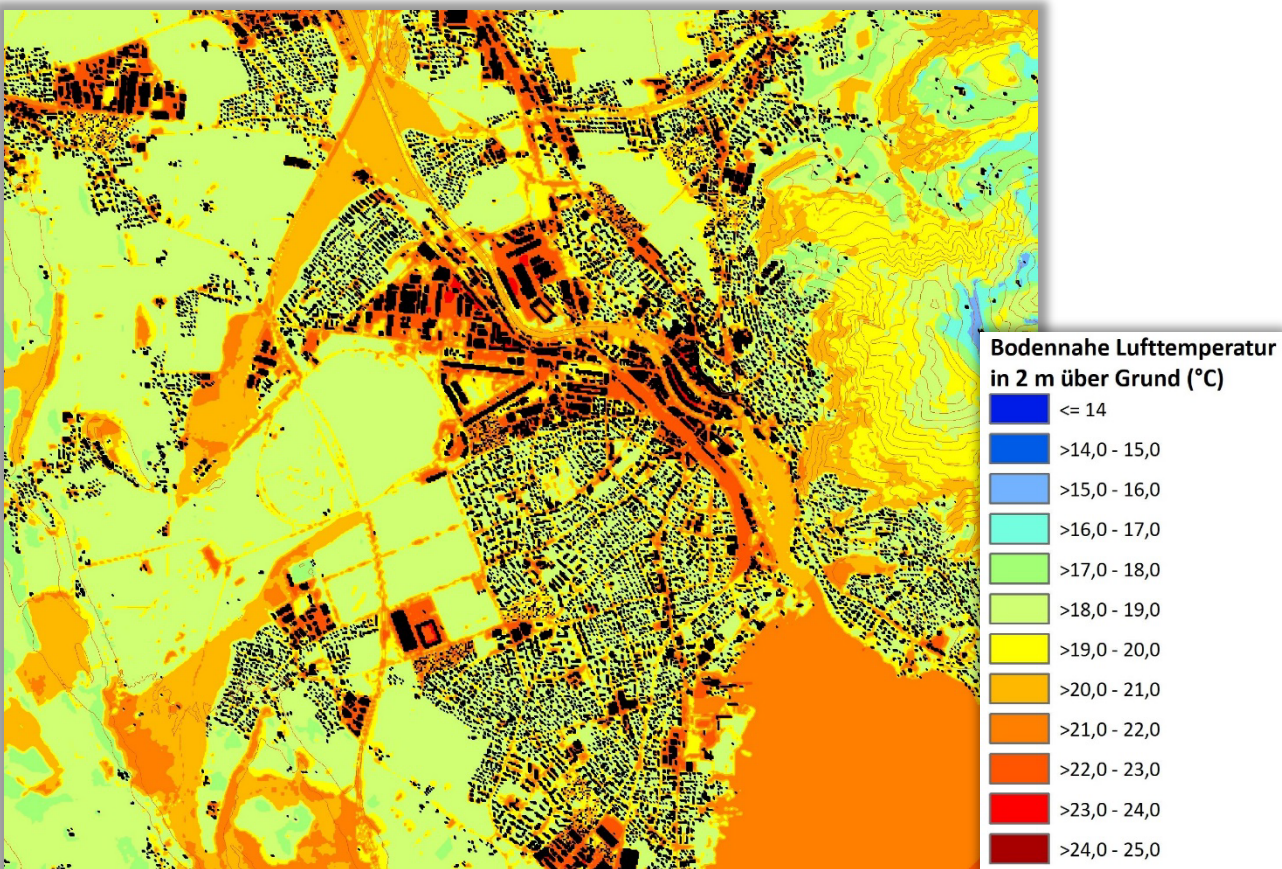
Abb. 4.5: Temperaturfeld Zukunftsszenario im Bereich Bern zum Zeitpunkt 4 Uhr morgens (2m ü. Grund)
