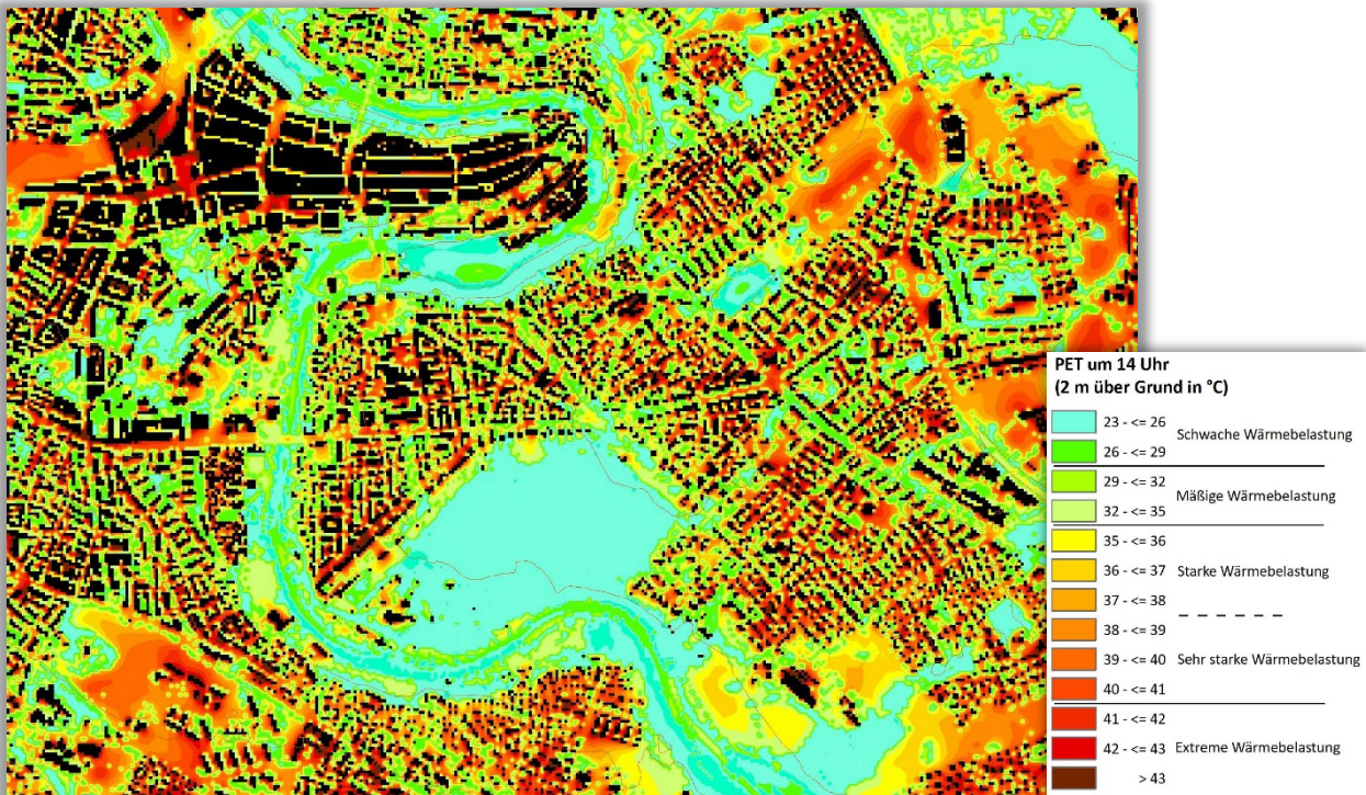
Abb. 4.8: PET Gegenwart im Bereich Bern zum Zeitpunkt 14 Uhr mittags (2m ü. Grund)
